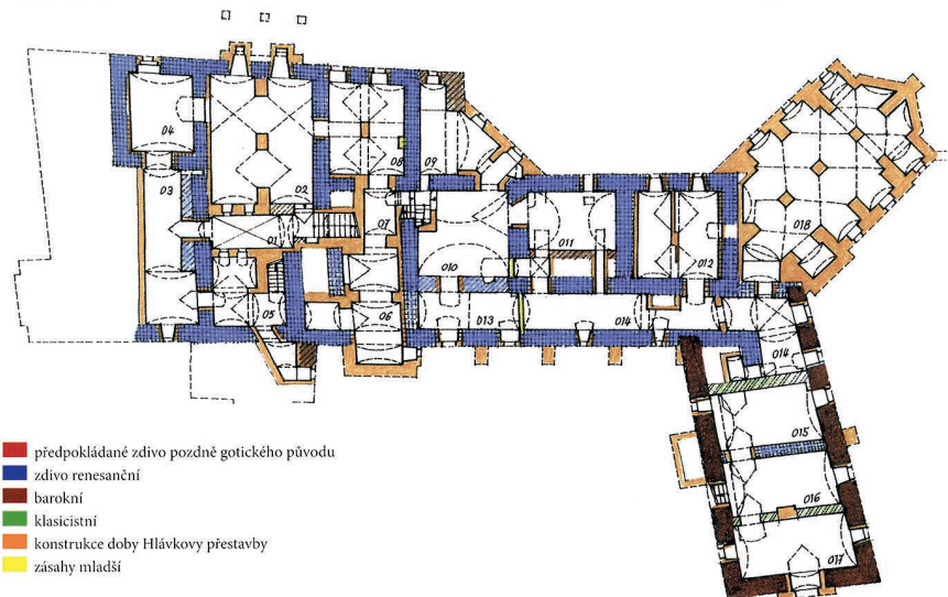
Sklepy zámku ve stavebně historické analýze, plán arch. Františka Kašičky
