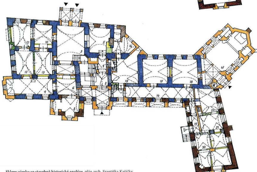
Sklepy zámku ve stavebně historické analýze, plán arch. Františka Kašičky
